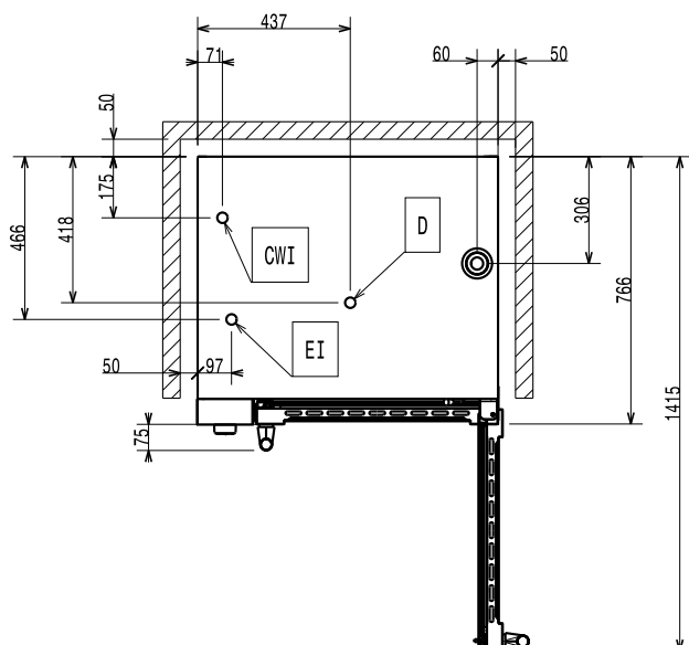
Boven aanzicht
